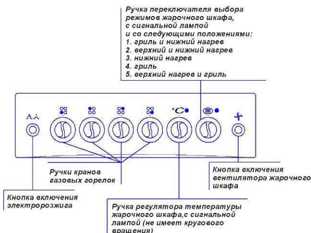
Рис. 11. Передняя панель плиты CGE-540 esWh
