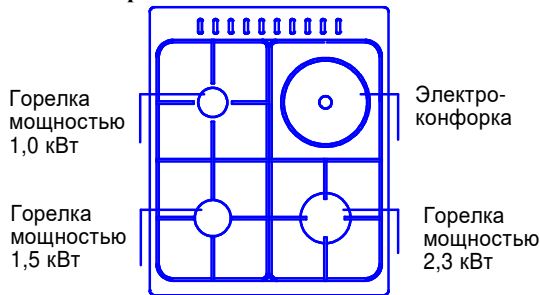
Рис. 14. Верхняя панель плит CGE-531 ecWh
