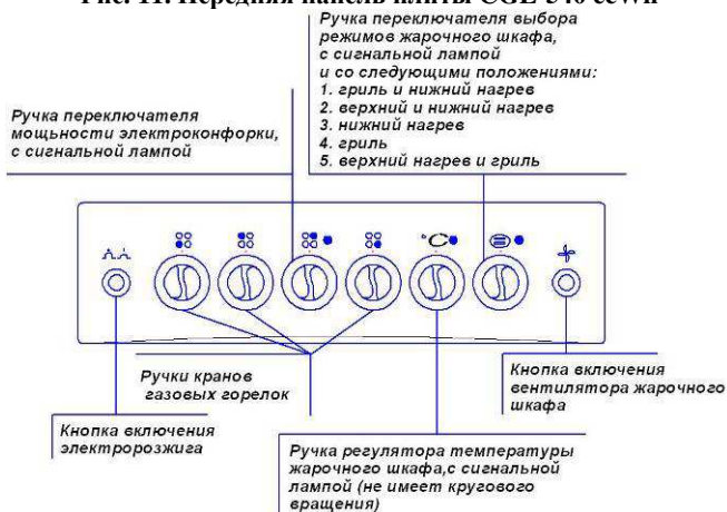
Рис. 12. Передняя панель плит CGE-531 esWh
