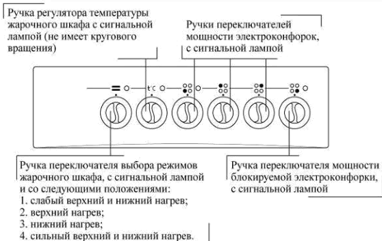
Рис. 8 Передняя панель плиты CSE-54 Wh, CSE-54 Bk
